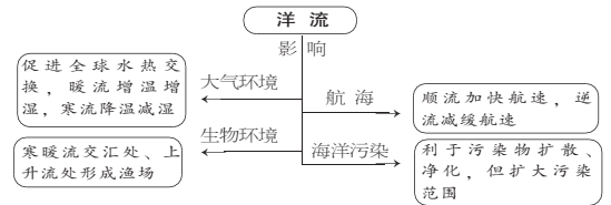
图 3 洋流对地理环境的影响
